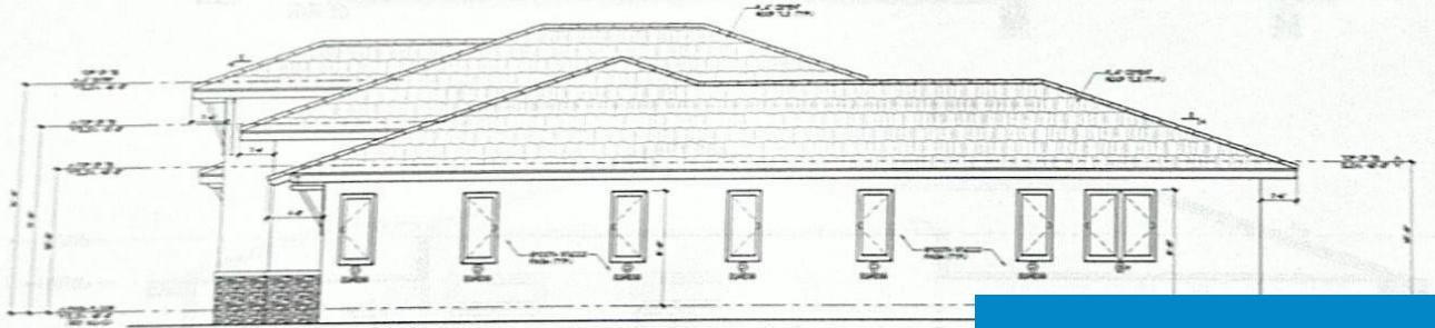
RIGHT ELEVATION
